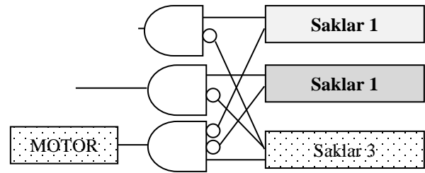
Gambar 11. Rangkaian Logika untuk Penerangan dengan Lintasan Segitiga
