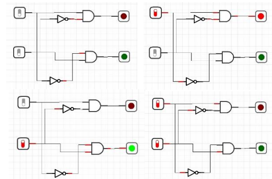
Gambar 12. Simulasi Rangkaian untuk Penerangan dengan Lintasan Garis Lurus
