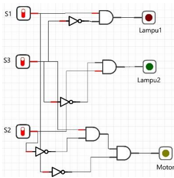
Gambar. 14. Simulasi Saklar saat Ditekan Bersamaan
