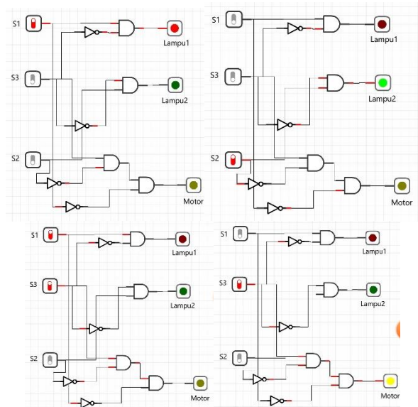
Gambar 13. Simulasi Rangkaian untuk Penerangan dengan Lintasan Segitiga
