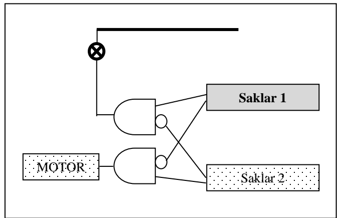
Gambar. 10. Rangkaian Logika untuk Penerangan dengan Lintasan Garis Lurus
